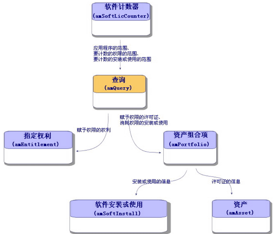
图形 8.3. 计数器、权利和资产组合项之间的链接
