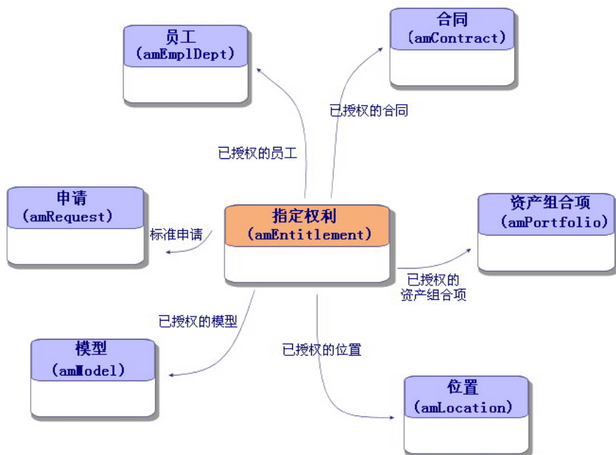
图形 8.2. 指定权利涉及的表
