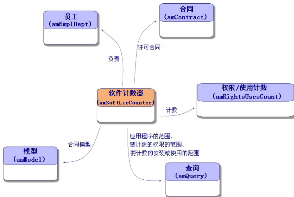
图形 8.1. 链接到计数器的表
