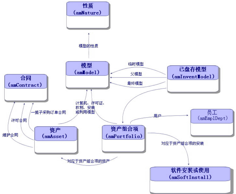
图形 2.1. 物理数据模型
