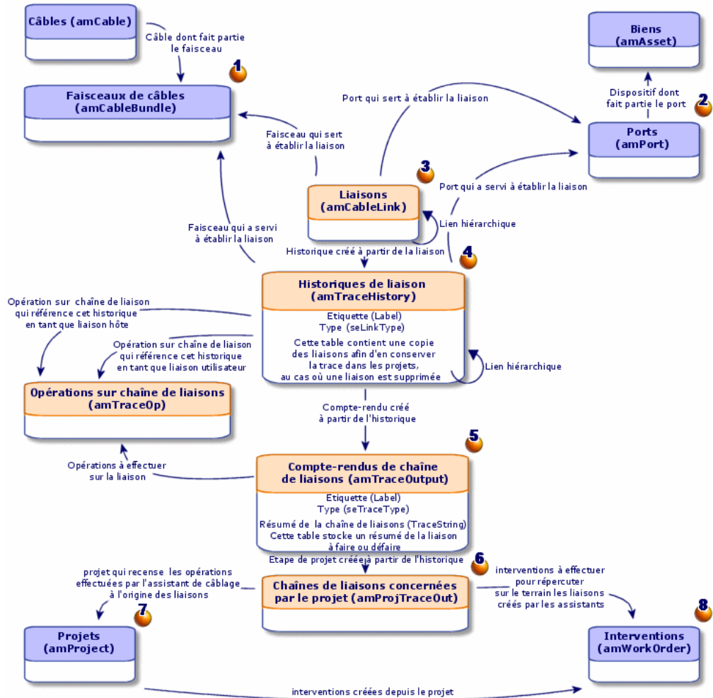
Figure 5.9. Liaisons - modèle de données détaillé
