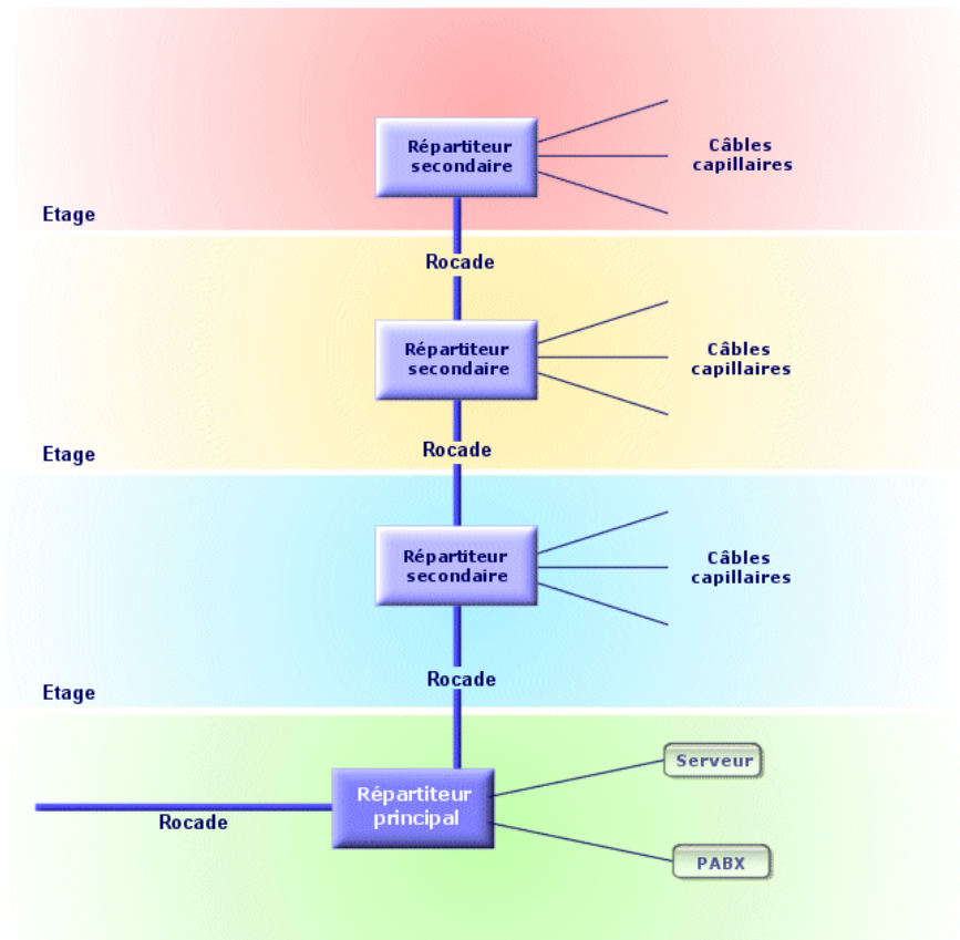
Figure 8.10. Distribution capillaire d'un réseau câblé - représentation
