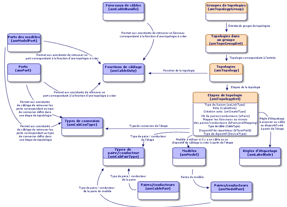
Figure 3.9. Topologies - modèle de données
