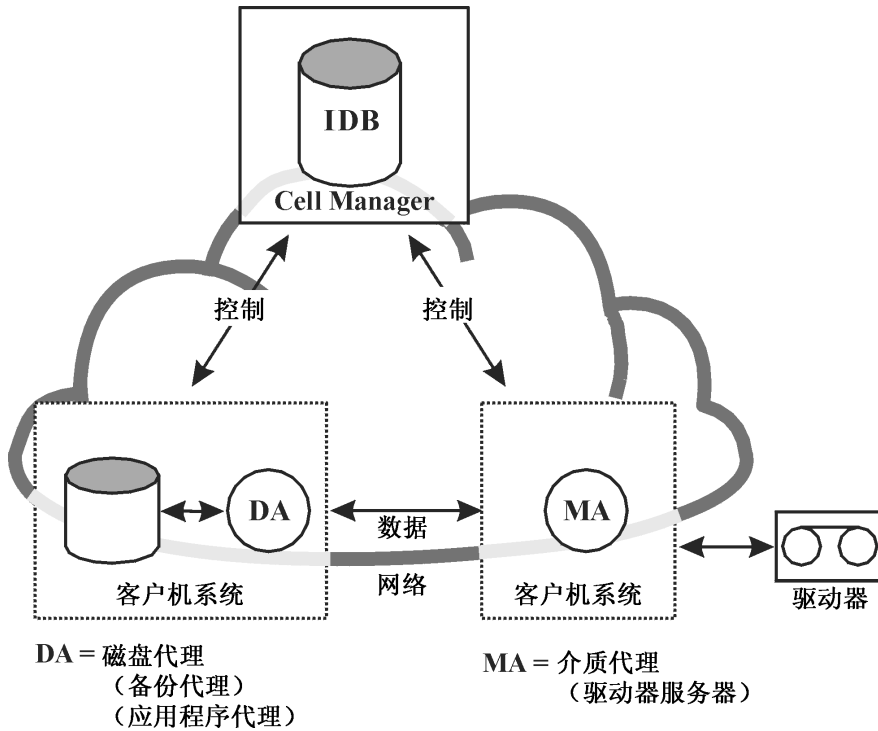
图 6 备份或恢复操作
