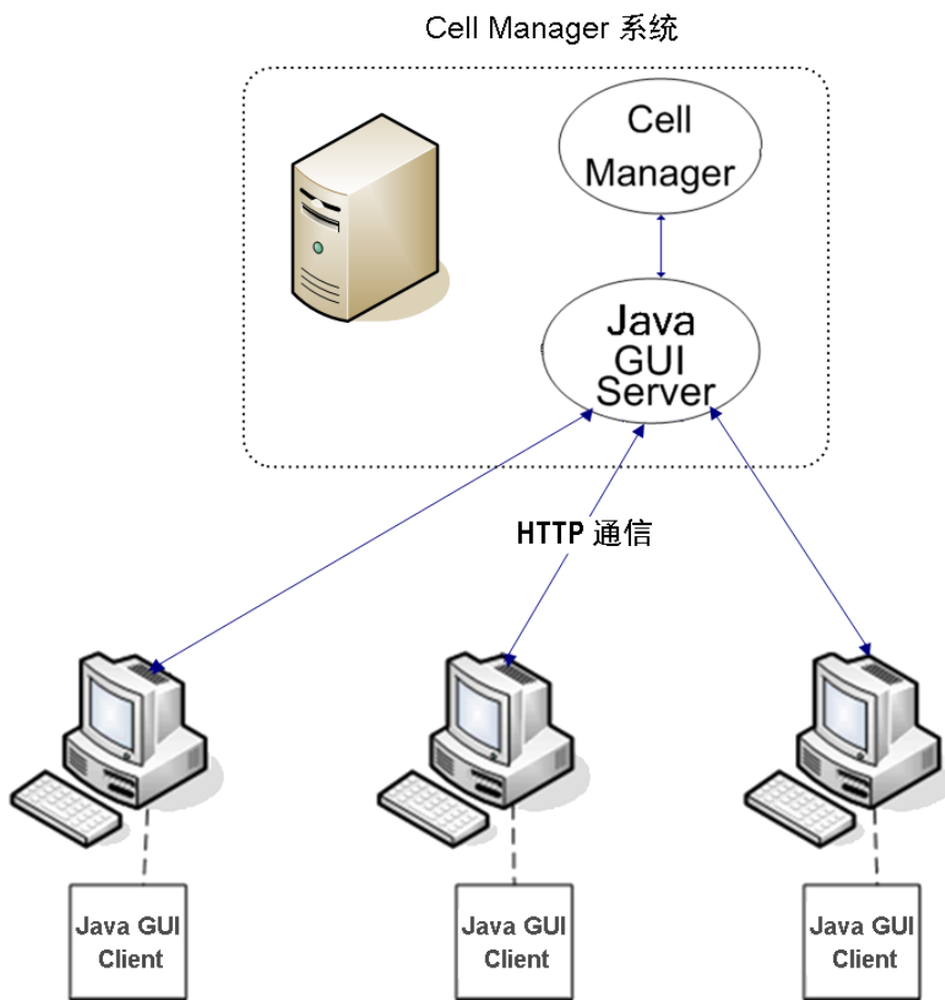
图 16 Data Protector Java GUI 架构
