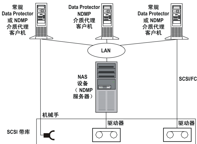
图 50 共享 SCSI 带库 (机械手与 Data Protector 客户机系统相连接)
