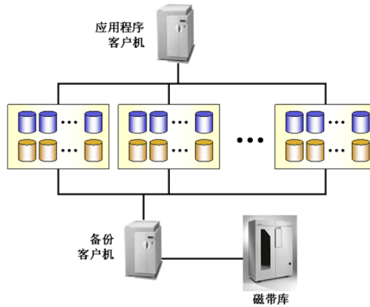
图 79 多个磁盘阵列 - 双主机
