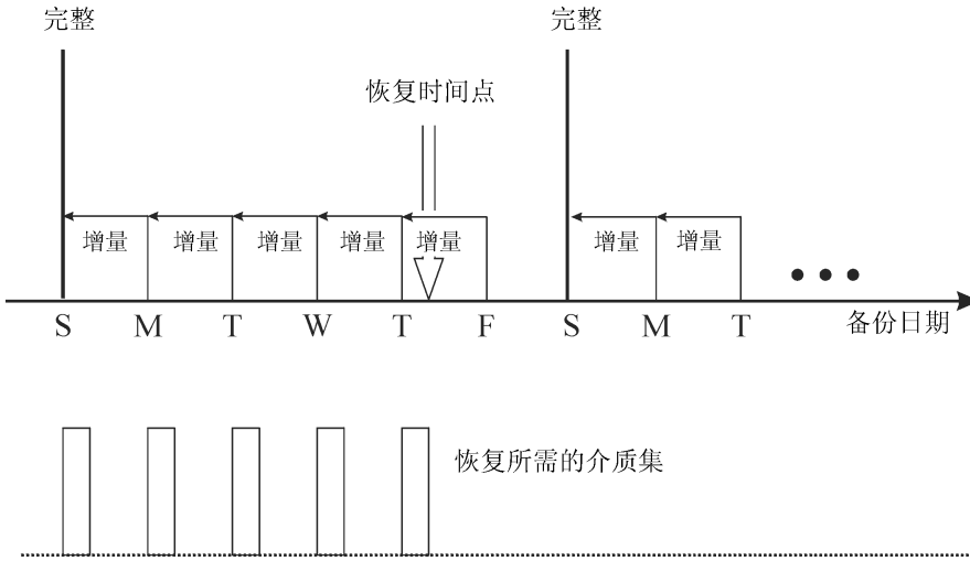
图 30 完整备份加每日简单增量备份
