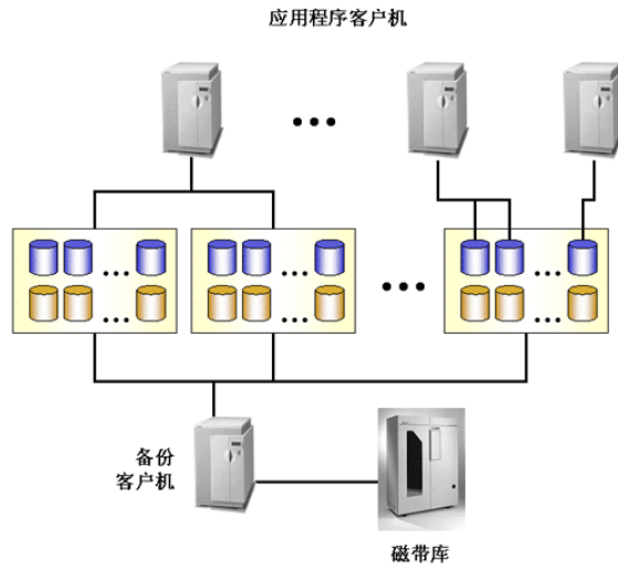
图 80 多台应用程序主机 - 单台备份主机
