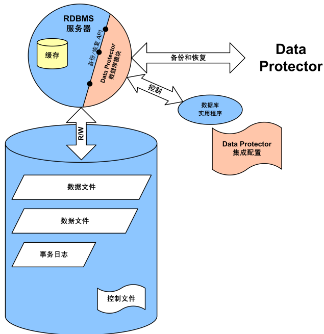
图 66 与数据库集成的 Data Protector
