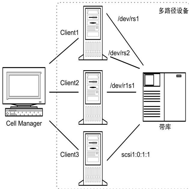
图 55 多路径配置示例
