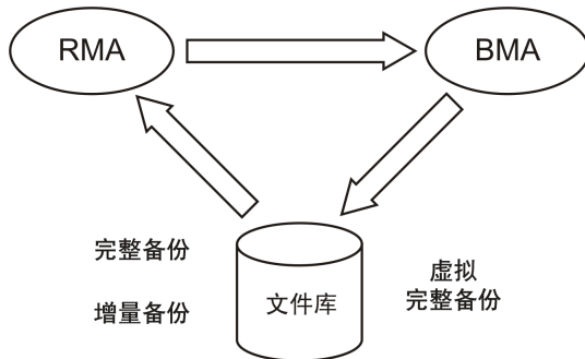
图 68 虚拟完整备份
