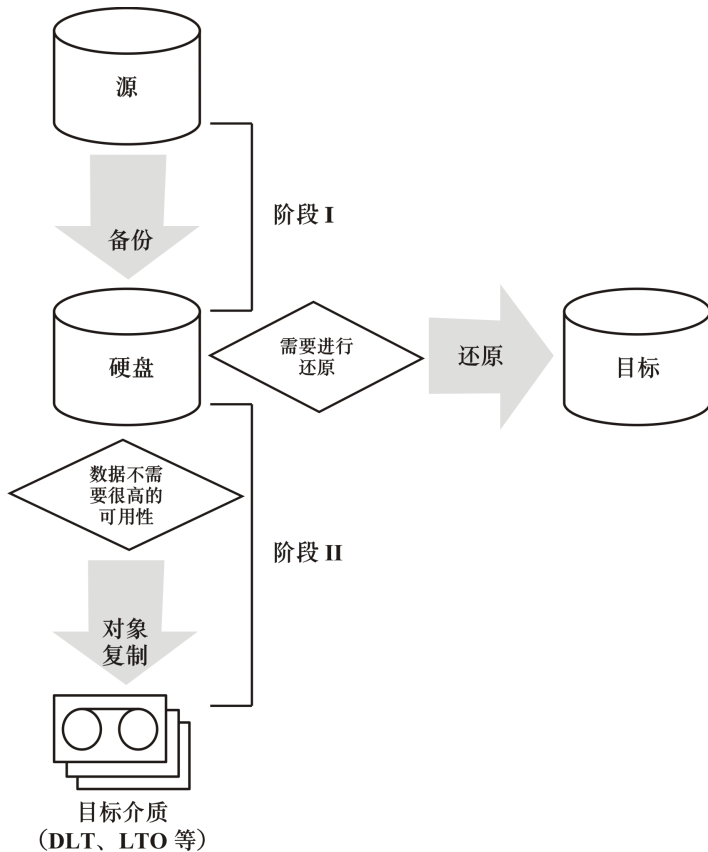
图 36 磁盘分段的概念
