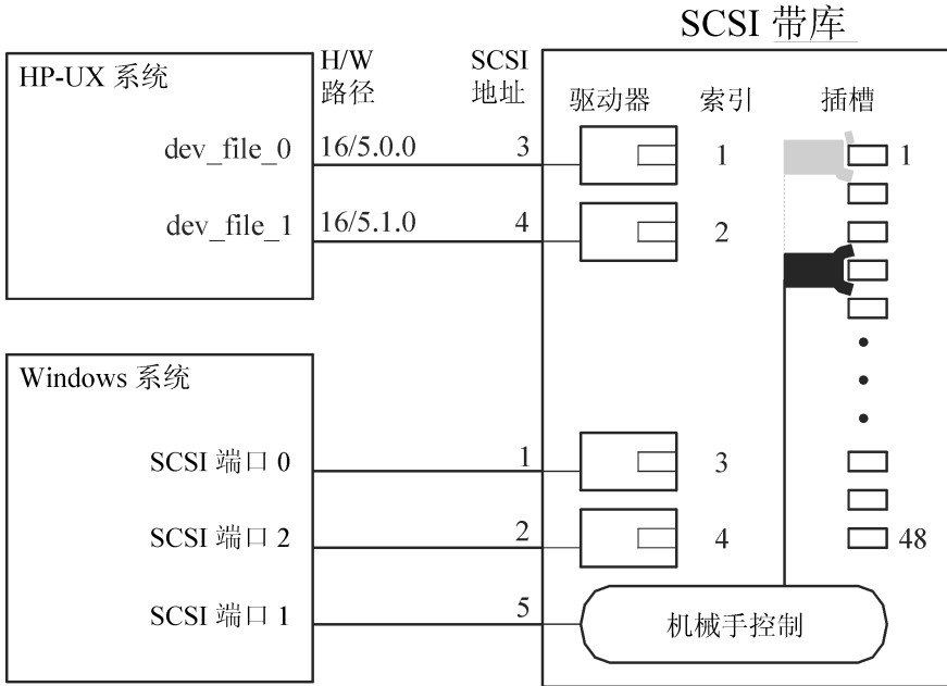
图 49 将驱动器与多个系统相连接
