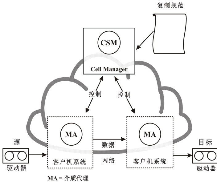
图 64 对象复制会话信息流
