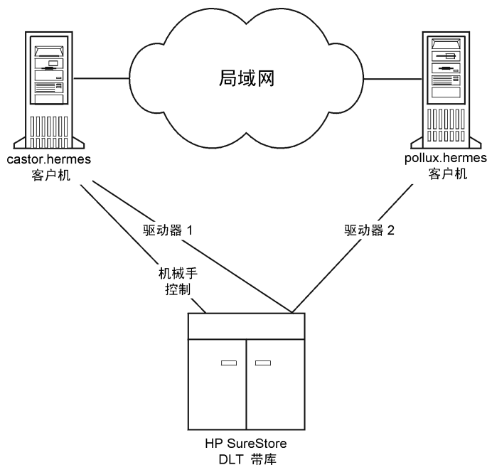
图 56 间接带库访问
