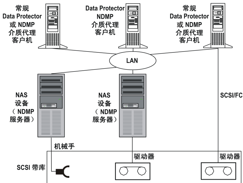
图 51 共享 SCSI 带库（机械手与 NDMP 服务器相连接）
