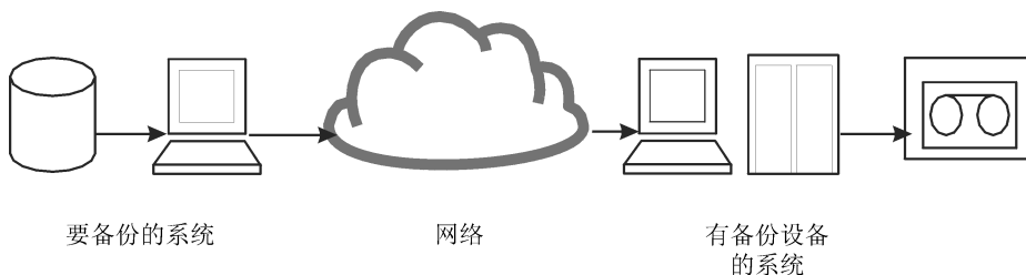
图 4 网络备份
