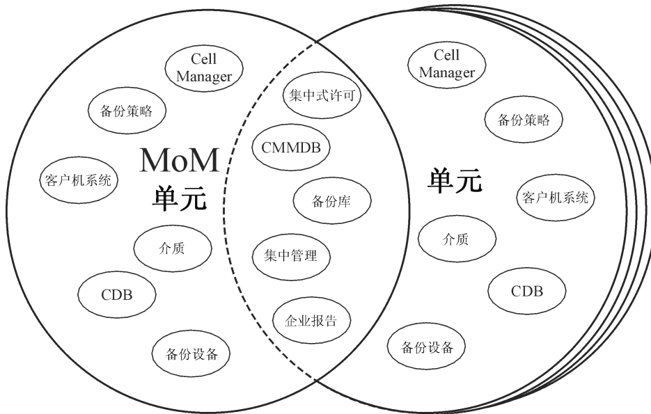
图 11 Manager-of-Managers 环境
