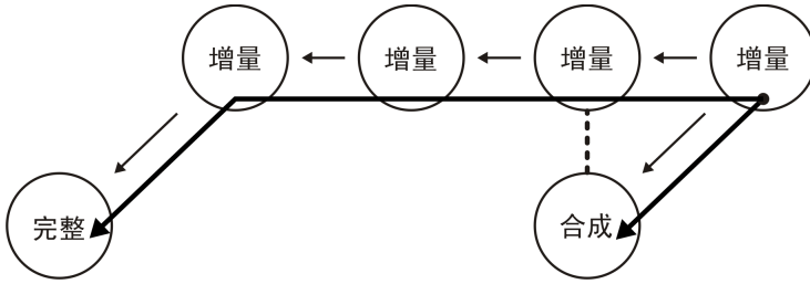
图 70 合成备份
