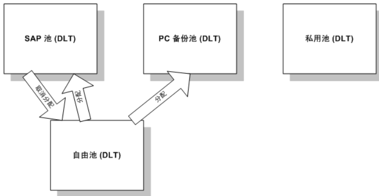
图 38 自由池
