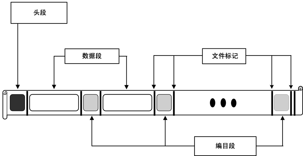
图 47 数据格式
