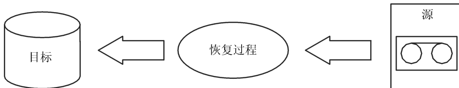
图 3 恢复过程
