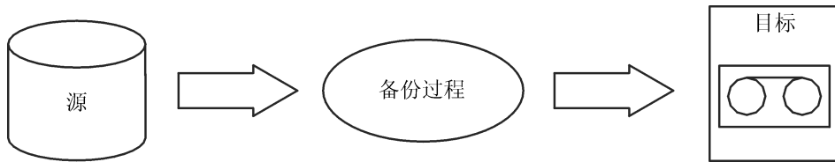
图 2 备份过程
