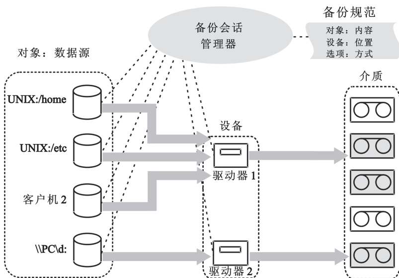
图 29 备份会话
