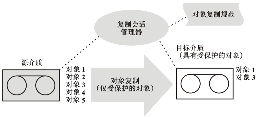
图 34 释放介质
