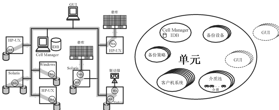
图 5 Data Protector 单元（物理视图和逻辑视图）
