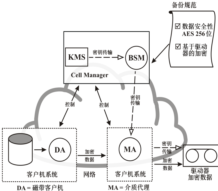
图 18 使用 AES 256 位加密和基于驱动器加密的备份会话
