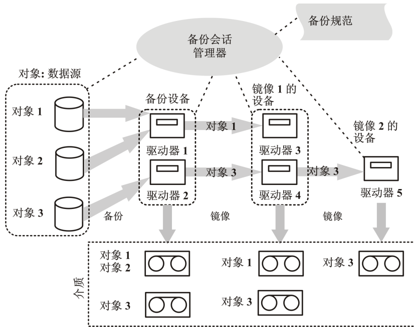
图 37 对象镜像
