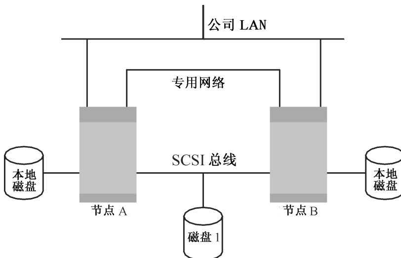
图 21 典型群集
