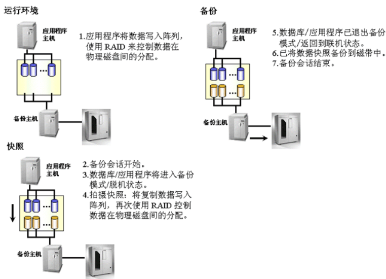
图 77 快照备份
