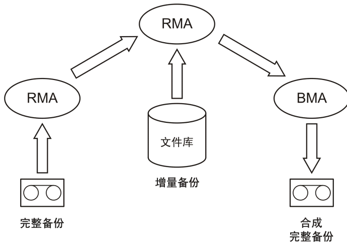
图 67 合成备份
