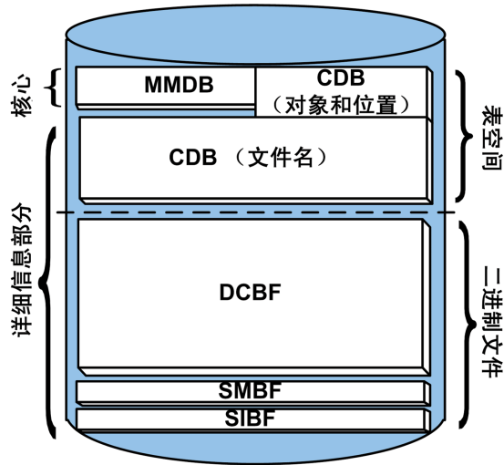
图 58 IDB 部分
