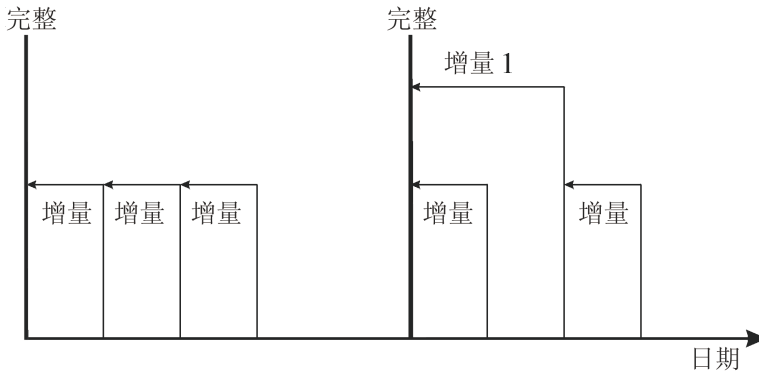
图 25 增量备份
