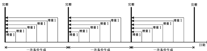
图 93 备份生成
