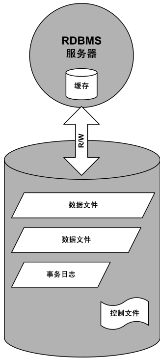
图 65 关系数据库
