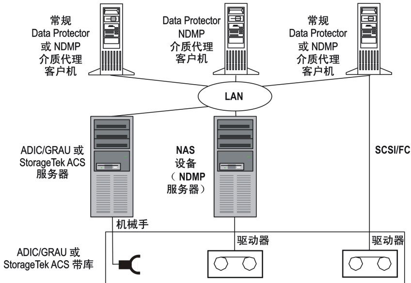
图 52 共享 ADIC/GRAU 或 StorageTek ACS 带库
