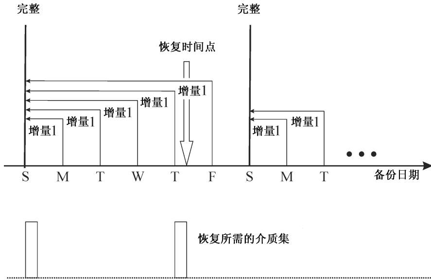
图 31 完整备份加每日一级增量备份
