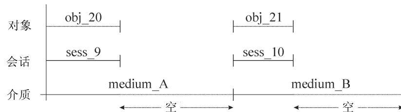
图 46 每个对象写入单个介质
