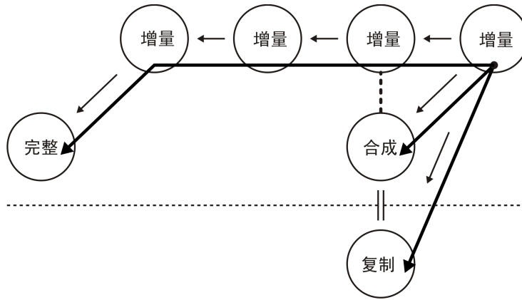
图 72 合成备份和对象复制
