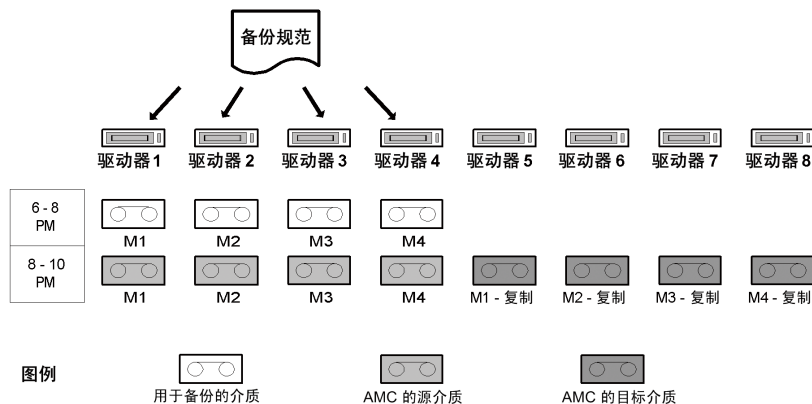
图 97 完整数据库备份和自动介质复制
