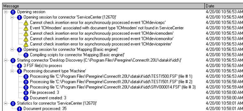
図 5.1. Connect-Itログ
